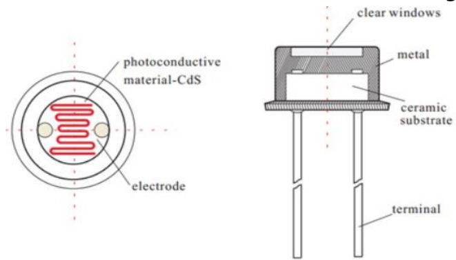
光敏电阻结构图 ( Photo resistor structure diagram )
