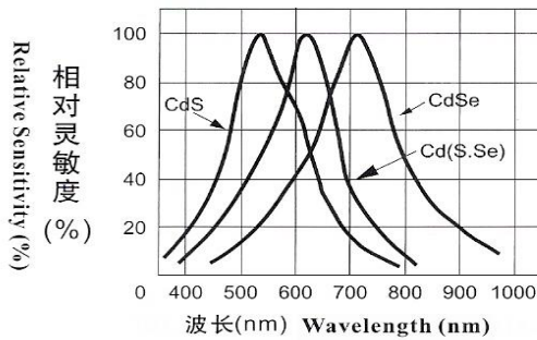
光谱响应特性 Spectral Response
