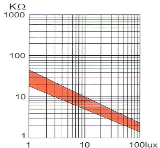
照度-电阻特性
