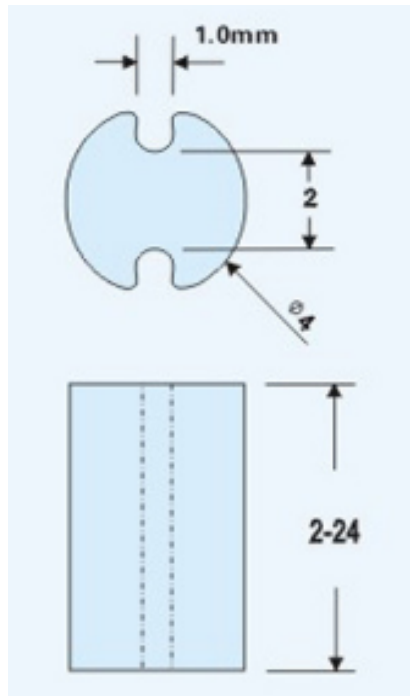
尺寸图
