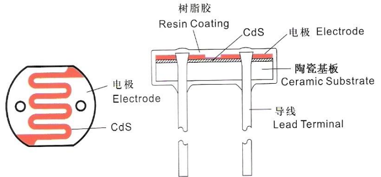
光敏电阻结构图 ( Photo resistor structure diagram )
