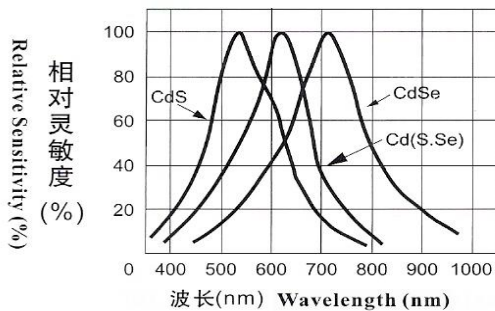
光谱响应特性 Spectral Response
