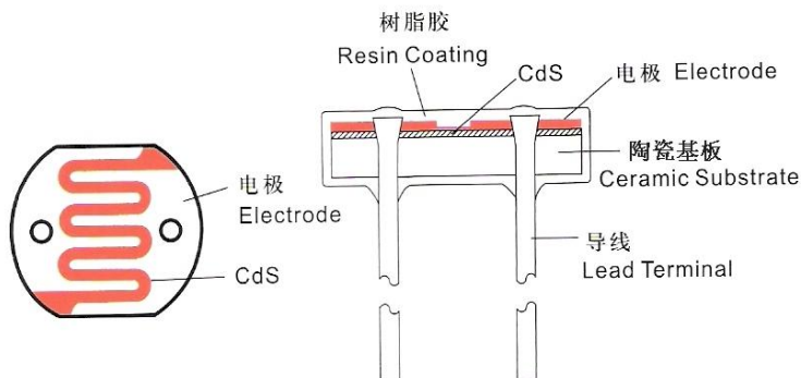
光敏电阻结构图 ( Photo resistor structure diagram )
