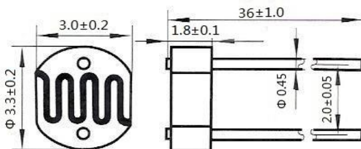
外形尺寸图 ( 单位 : mm )
