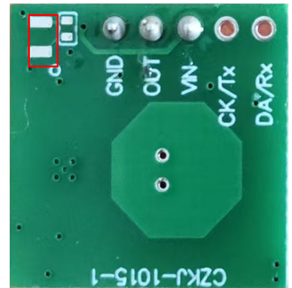
图6 光敏位置（预留）
