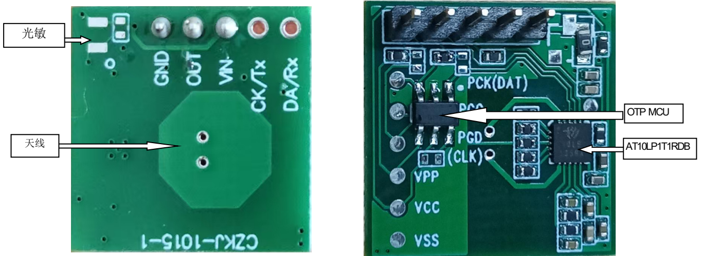
图1 CZKJ-1015-1 模块实物图
