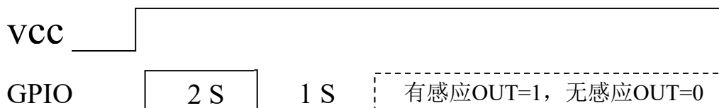
图7模块上电时序图
