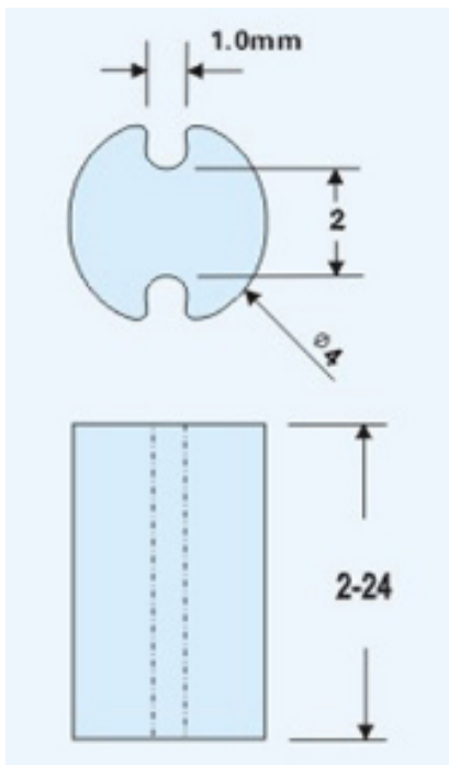
尺寸图
