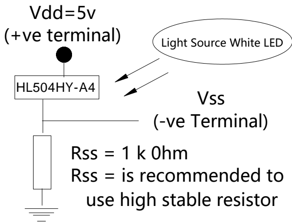
电路原理图
